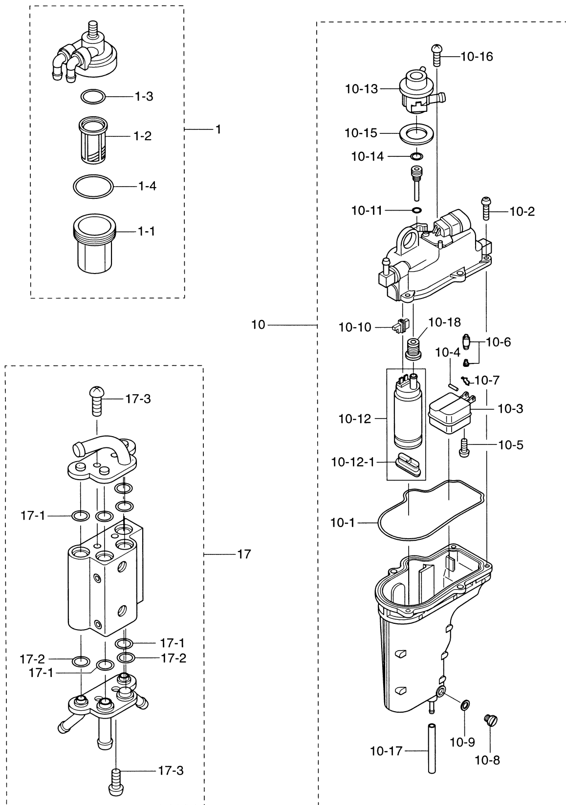
フュエルポンプ、フュエルレール&ペーパーセパレータ Fig. 5 FUEL PUMP, FUEL RAIL & VAPOR SEPARATOR
