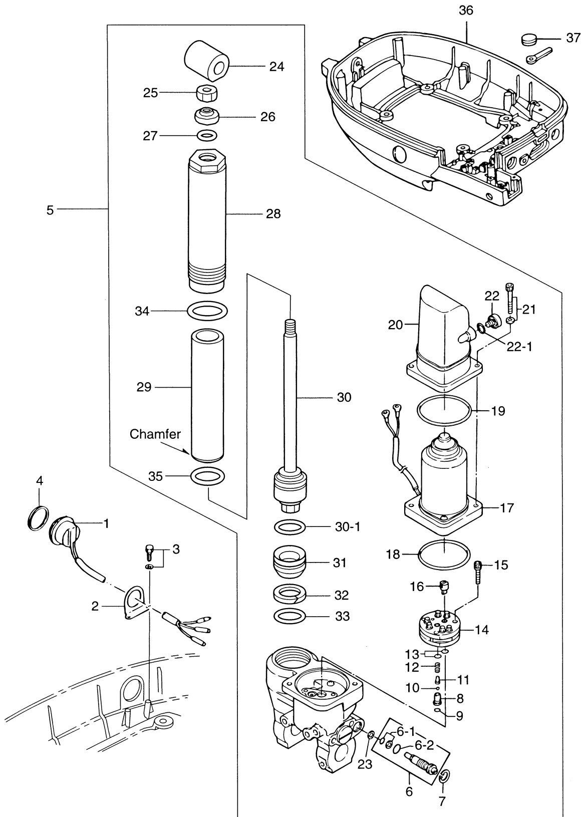
パワートリム&チルト POWER TRIM & TILT Fig. 21
