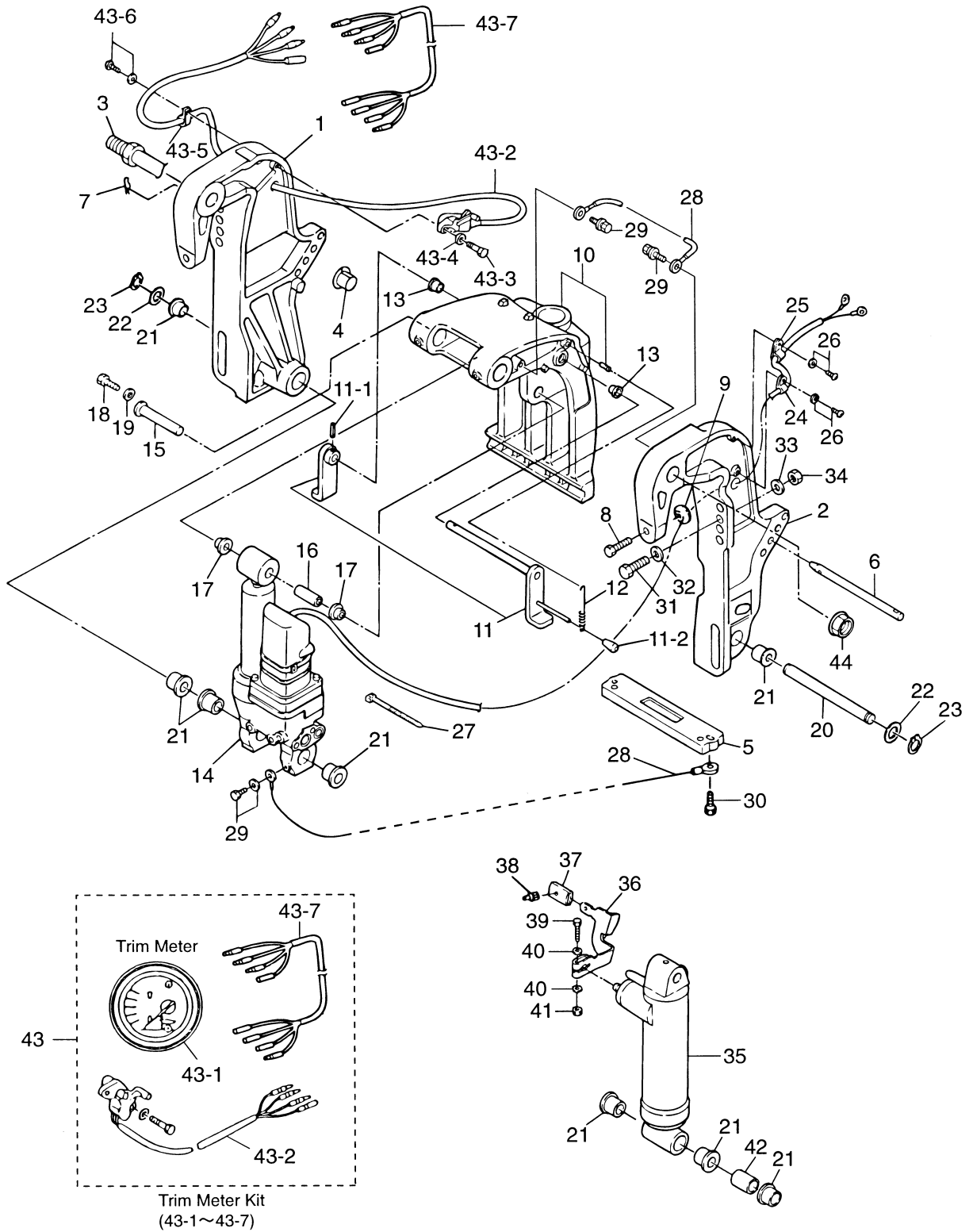
ブラケット、PTT & ガスアシスタント Fig. 20 BRACKET, PTT & GAS ASSISTANT
